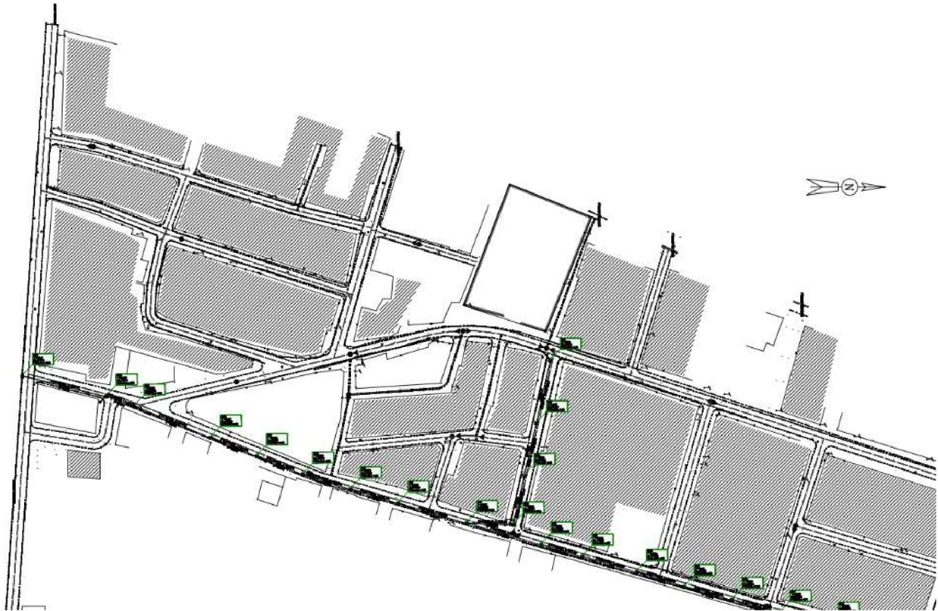
Figure 7:Tracé En Plan des Collecteurs Partie 01
