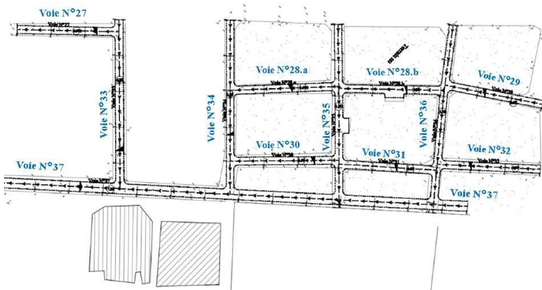
Figure 11: Plan des Voiries_ partie03
